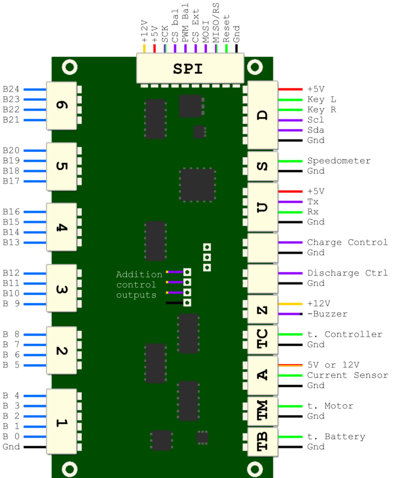
Розпінування сигнальної частини пристрою. Вид зверху.
