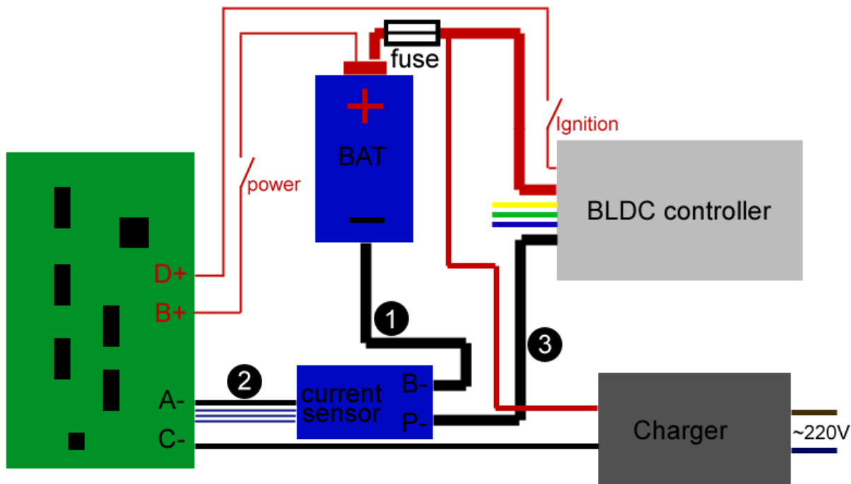
Базова схема та порядок підключення силових ліній, живлення і слабкострумowego запалювання (нижня плата)
